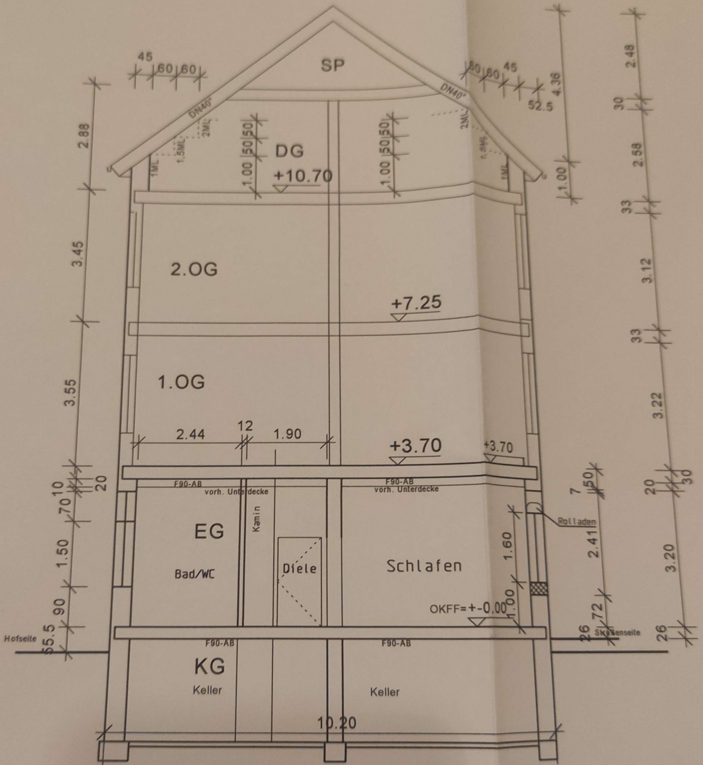
Schnitt A - A M 1:100
